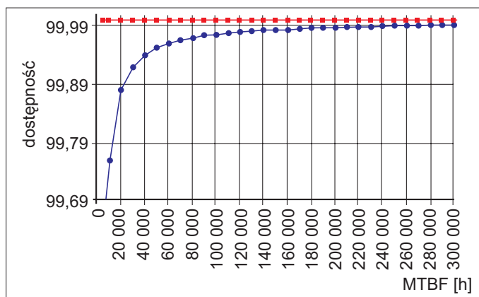
Rys. 1. Dostępność zasilania w funkcji współczynnika MTBF
